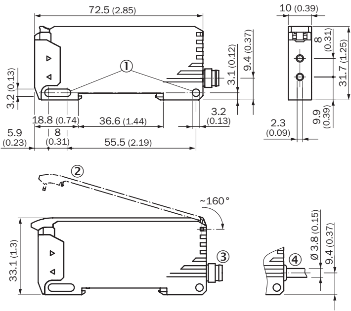
尺寸图 (尺寸单位: mm)
