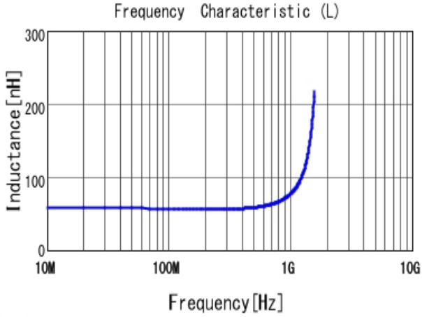
■ LQP03TN56NH02 L
