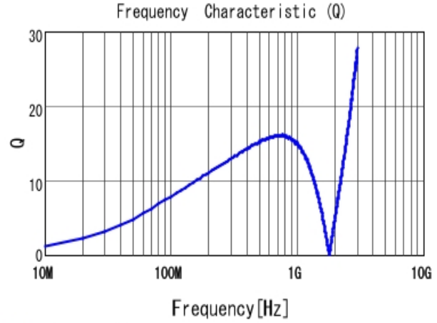
■ LQP03TN56NH02 Q
