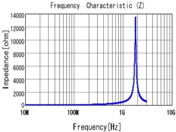
■ LQP03TN56NH02 |Z|
