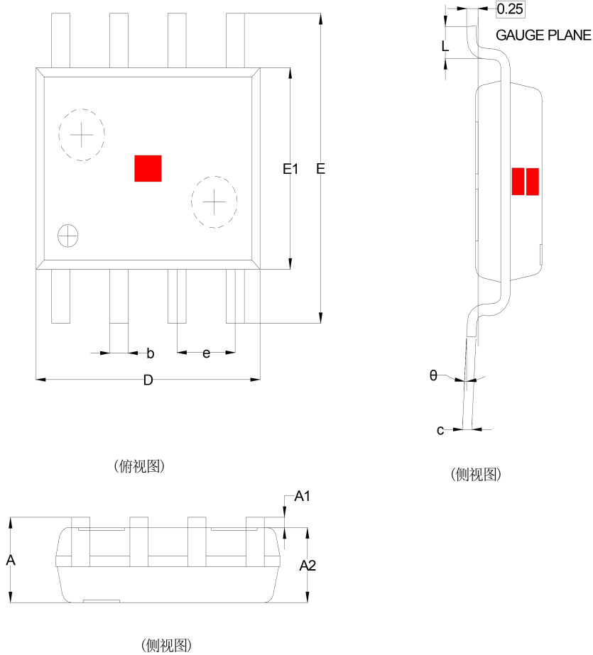
图示：SOP8 封装外形（单位：毫米）
