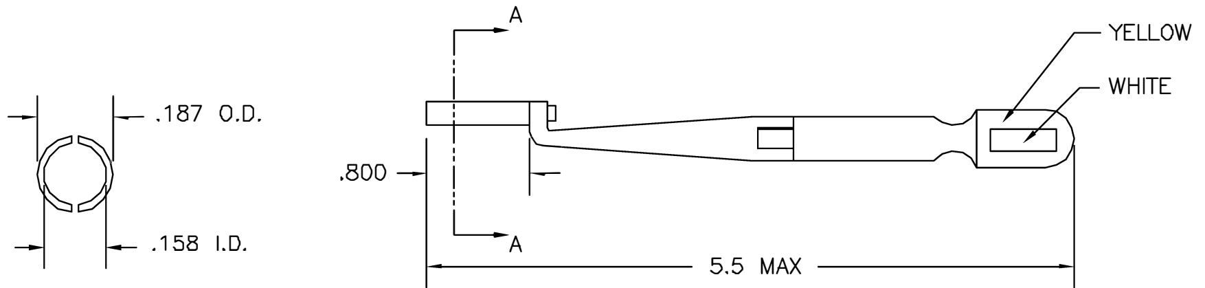
VIEW A-A
