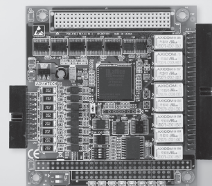
PCM-3761I
