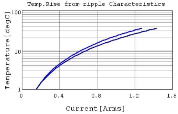
GRM033R61E224KE01 Temp.rise — 600kHz
