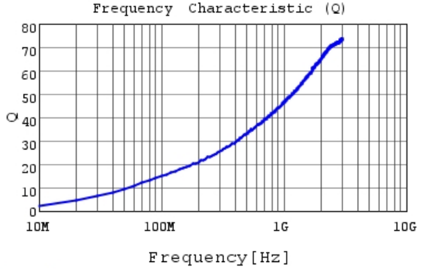
LQW15AN3N1B00 Q
