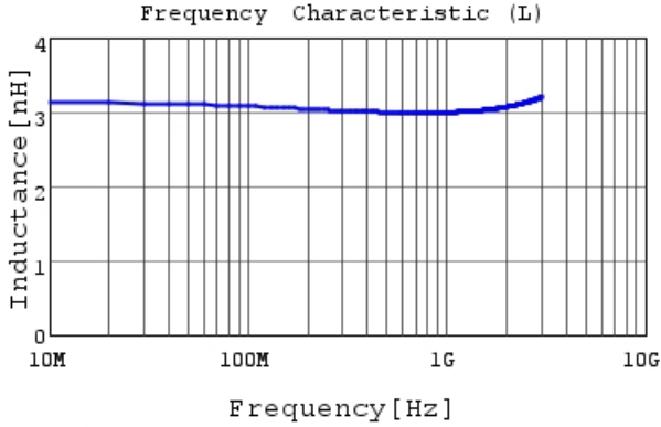
LQW15AN3N1B00 L
