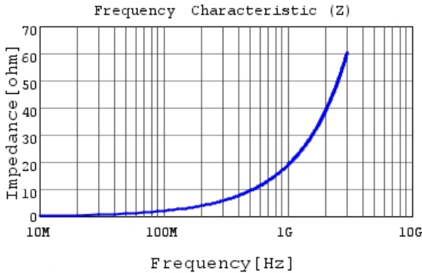
LQW15AN3N1B00 |Z|
