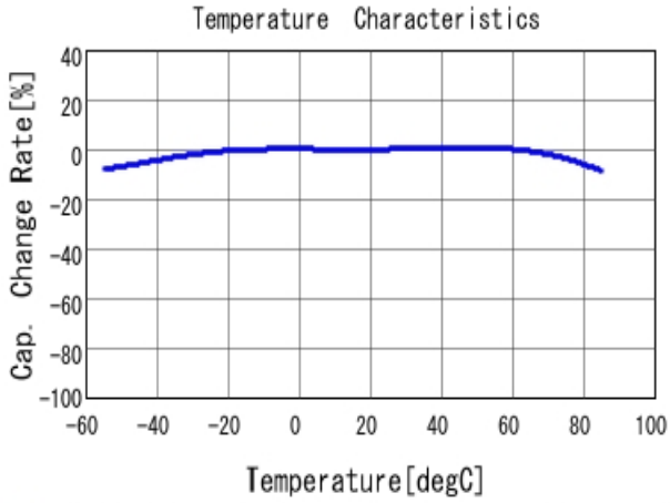
■ GRM033R61C104KE18 C-Temp. capchange, DCO. 0V, ACO. 5Vrm
