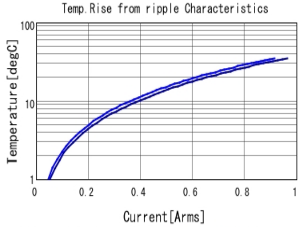
GRM033R61C104KE18 Temp. rise ■ 800kHz ■ 1MHz
