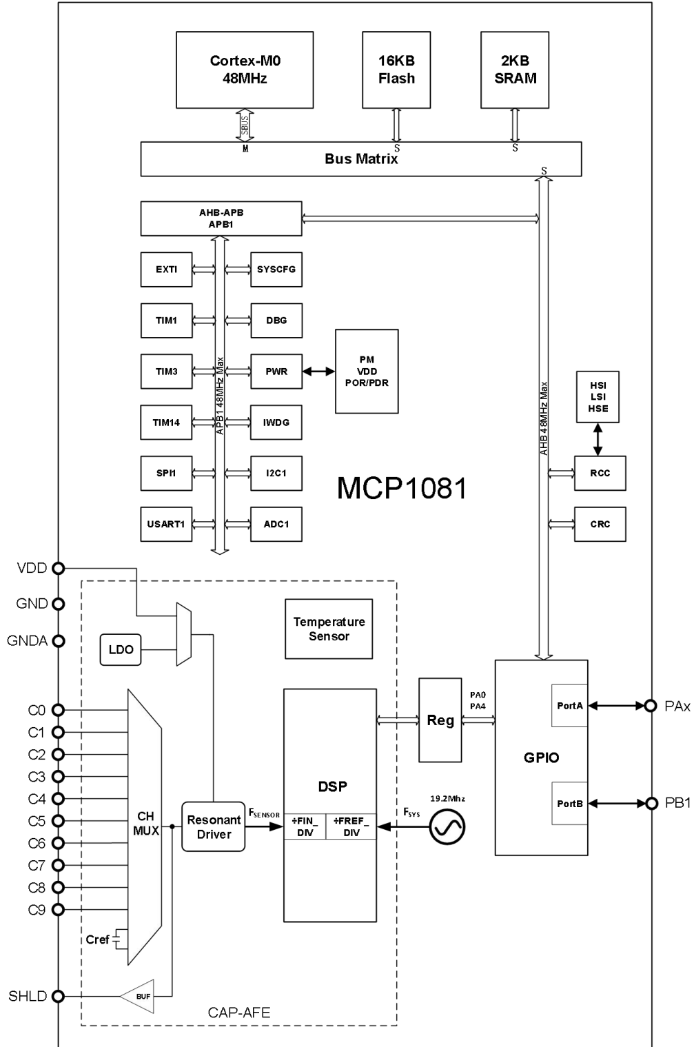
图 6.1 系统框图
