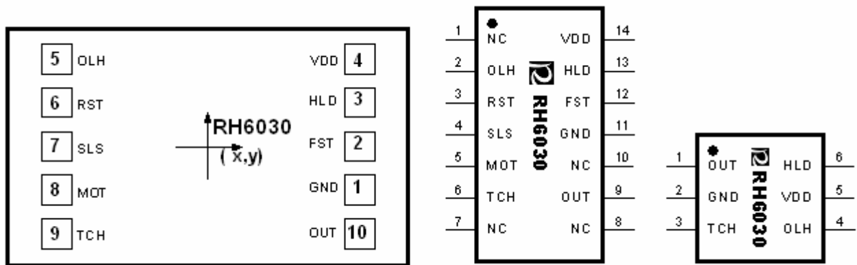
图 1 Die / SOP14/SOT23-6L 封装示意图
