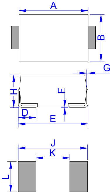
DO-214AC (SMA)
