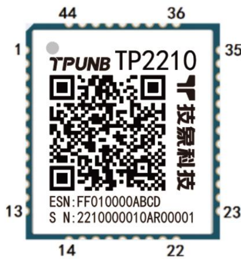
图 1 网关俯视图
