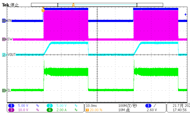
Figure 14. EN Toggle, IOU=3A
