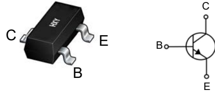
SOT-23
