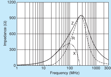
BLM15BX601SZ1
