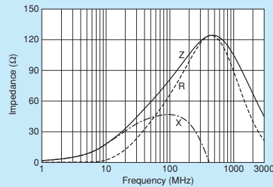
BLM15PX800SZ1
