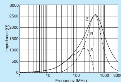
BLM18HD102SZ1/BLM18HD102SH1
