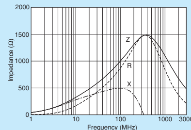
BLM18HG102SZ1/BLM18HG102SH1
