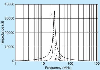
NFZ32BW221HZ10
