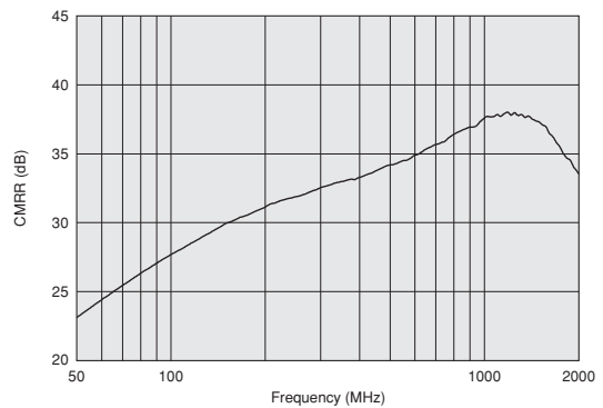
DXW21BZ7511T
