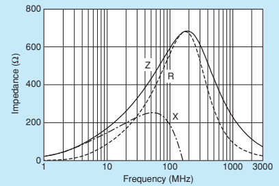
BLM18AG601SZ1/BLM18AG601SH1
