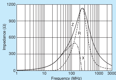
BLM18BD182SZ1/BLM18BD182SH1
