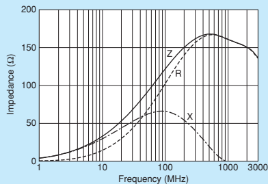
BLM15EG121SZ1
