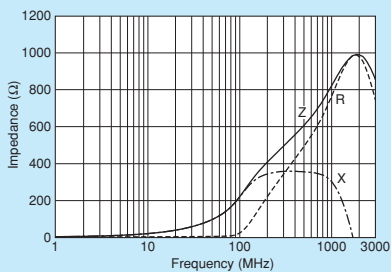
BLM15HB221SZ1
