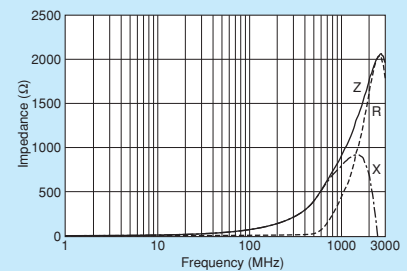
BLM15GA750SZ1
