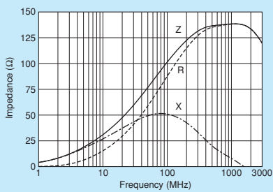
BLM18EG101TZ1/BLM18EG101TH1
