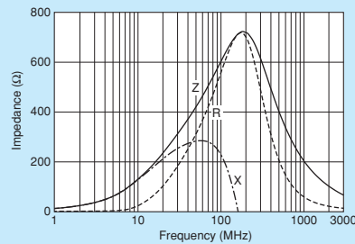
BLM15PX601SZ1
