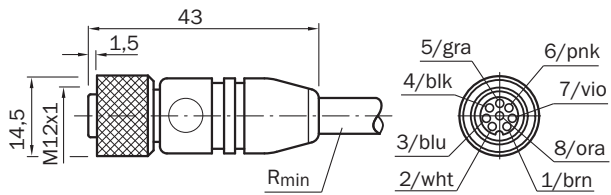
尺寸图 (尺寸单位: mm)
