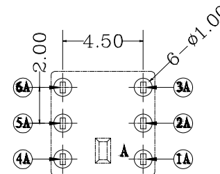
印刷电路板焊接处尺寸图
