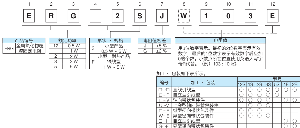
例2所示为额定功率2W小型金属氧化物覆膜固定电阻，其电阻值为10kΩ，电阻值容差为±5%，异型径向带状包装。
