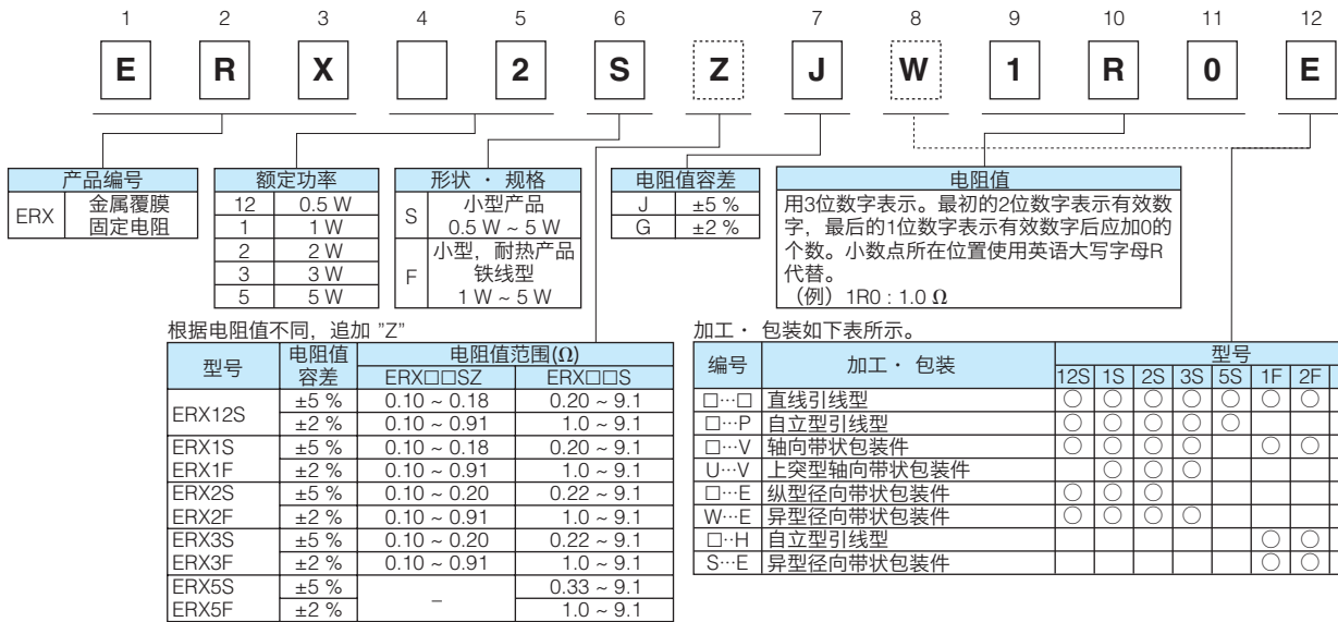
例1所示为额定功率2W的小型金属覆膜固定电阻，其电阻值为1.0Ω，电阻值容差为±5%，异型径向带状包装。
