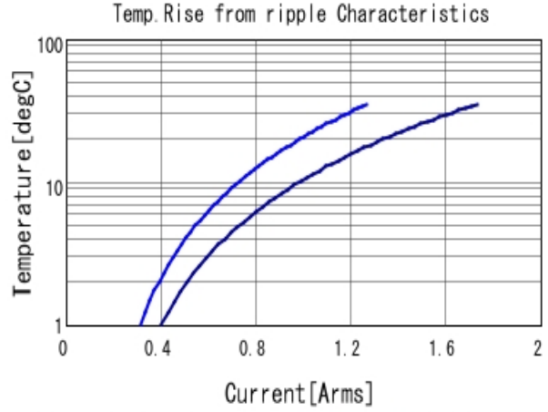
GRM188B31H104KA92 Temp. rise ■ 500kHz ■ 1MHz
