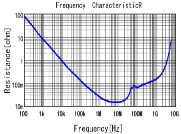
■ GRM188B31H104KA92 R DCOV, 20degC
