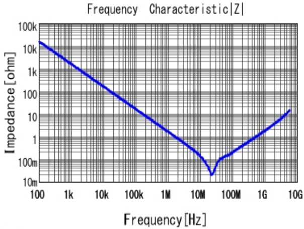
■ GRM188B31H104KA92 |Z| DCOV, 20degC
