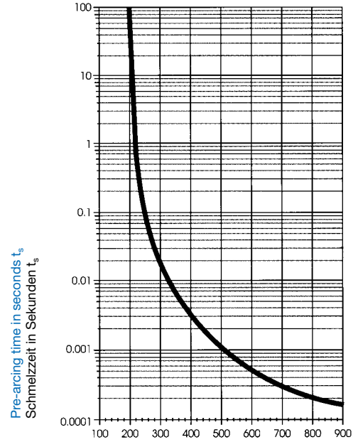
Percent of rated current I n / Prozent des Nennstromes I n
