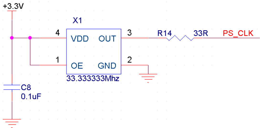
图 2-6-1 PS 部分的有源晶振
