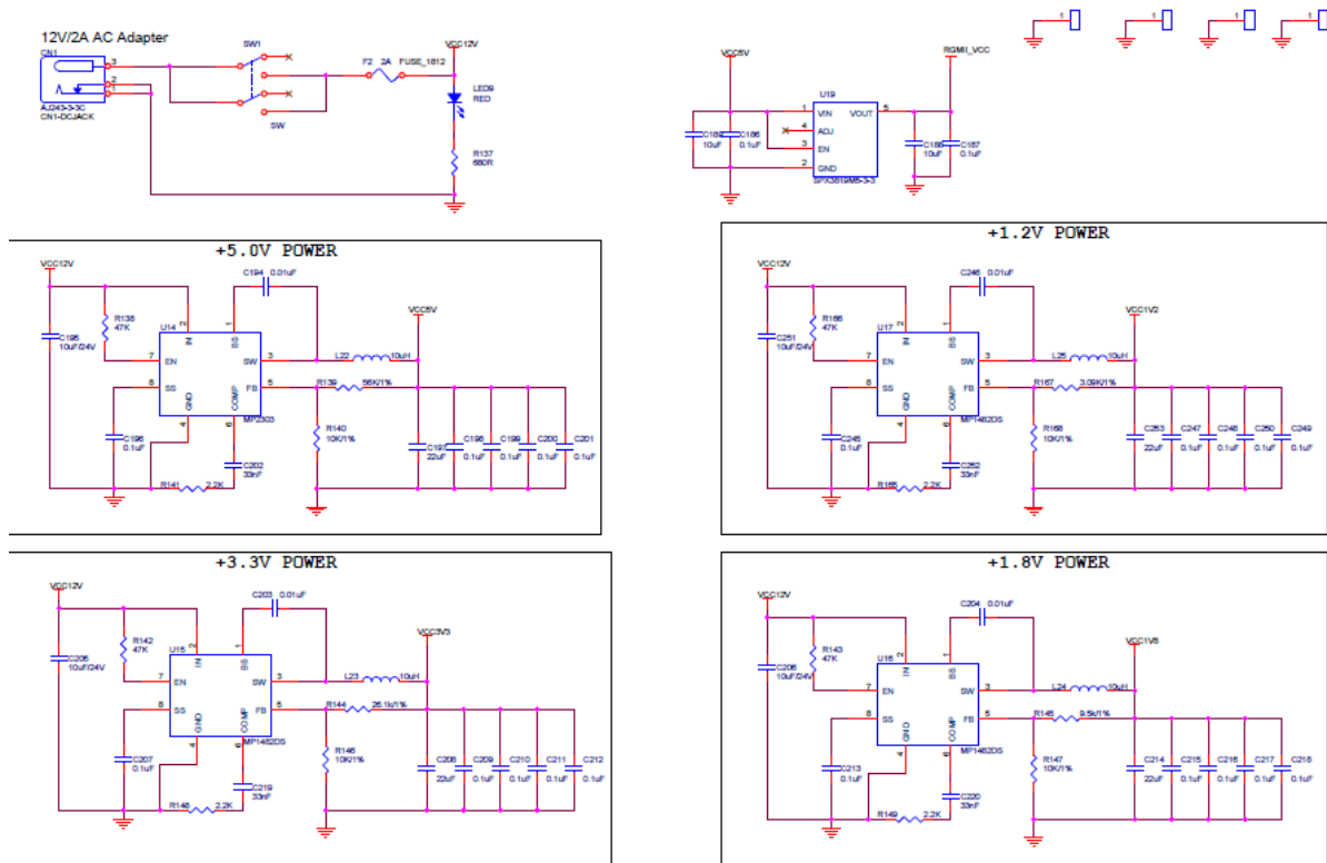
图 3-11-1 底板电源原理图
