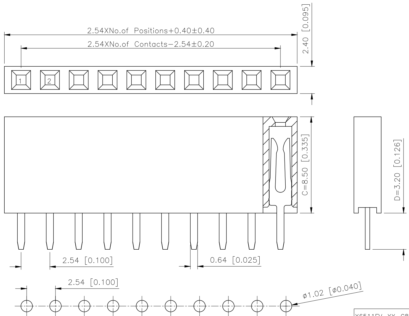
P.C.B LAYOUT
