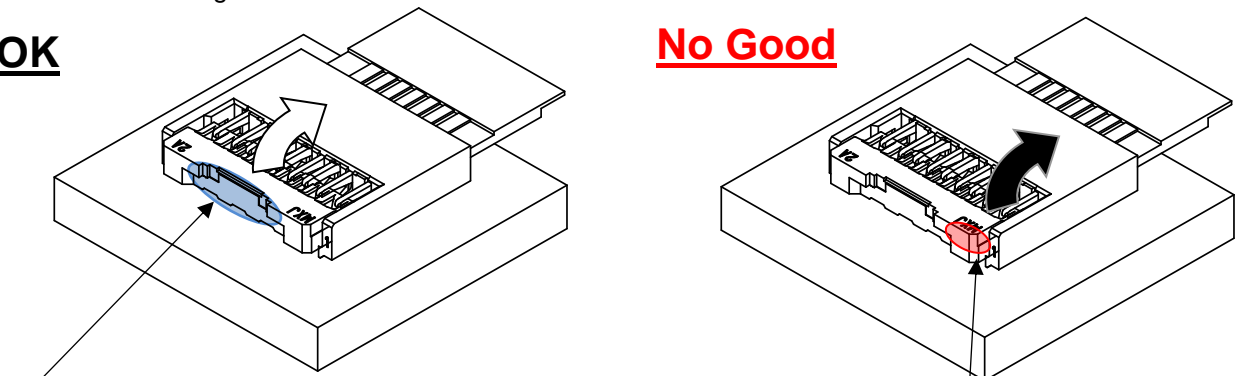
アクチュエータ下面中央部を操作 Push up the center bottom area of actuator
