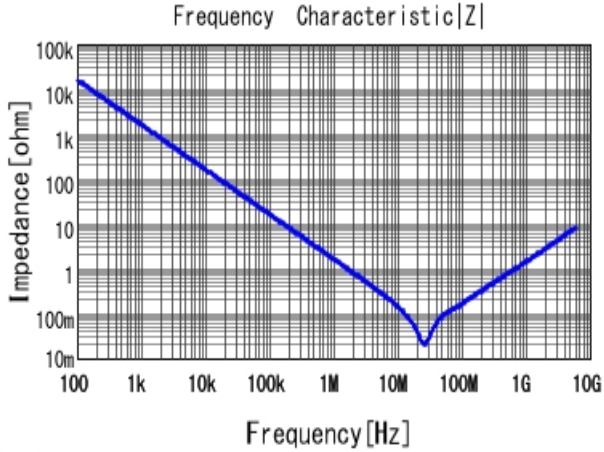
■ GRM155R61H104KE19 |Z| DCOV, 25degC
