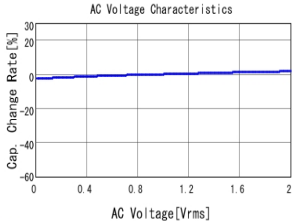
■ GRM155R61H104KE19 C-AC Voltage capchange, DCOV, 25.0d
