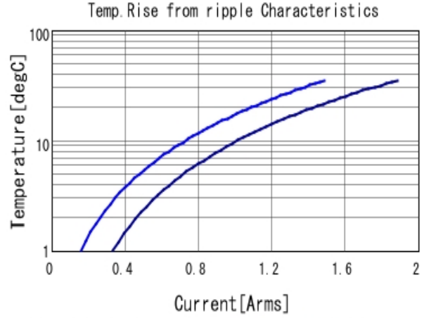
GRM155R61H104KE19 Temp. rise ■ 500kHz ■ 1MHz
