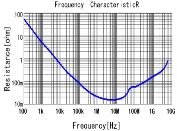
■ GRM155R61H104KE19 R DCOV, 25degC
