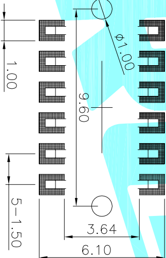
P.C.B layout
