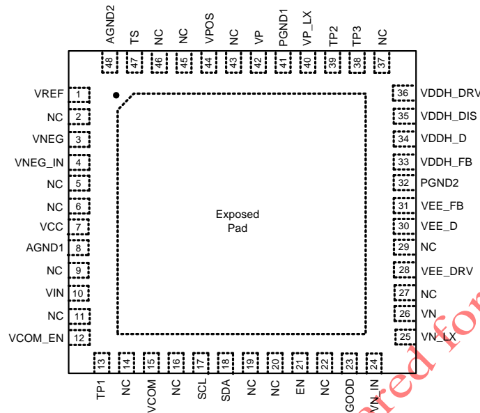
(QFN 6×6-48)
