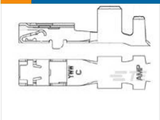
TE Part #1326030-3 2.8MM RECP,UNSEAL,14-16AWG
