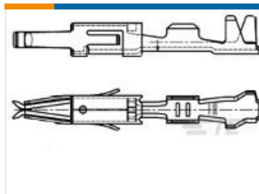
TE Part #2141900-3 MT 2,TERMINAL
