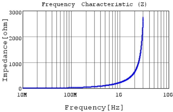
LQW18AS33NG0C |Z|
