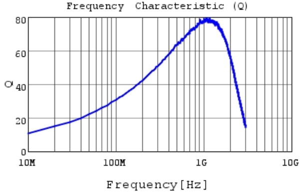
LQW18AS33NG0C Q
