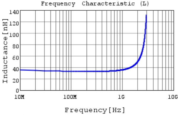
LQW18AS33NG0C L
