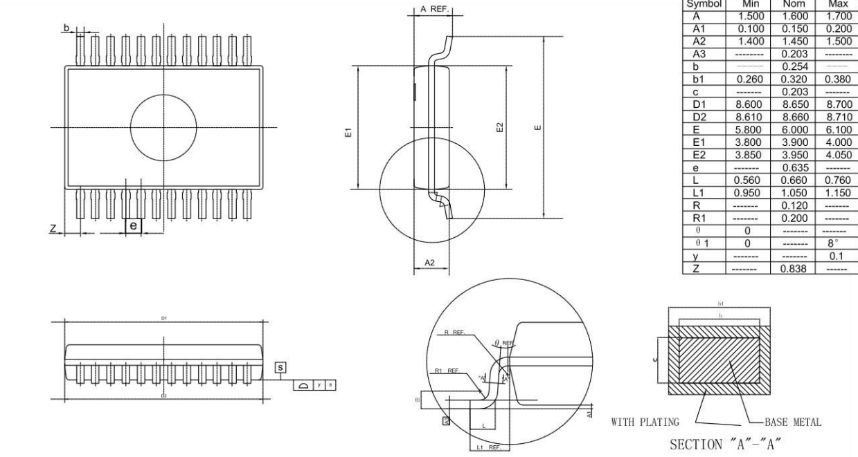
SSOP-24 (0.635mm) 外形图与封装尺寸
