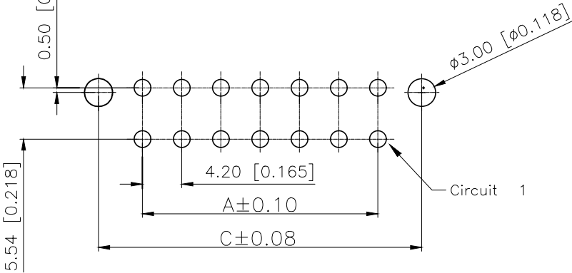
P.C.B Layout
