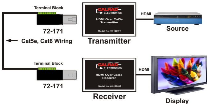
Calrad 40-1090 HDMI Baluns
