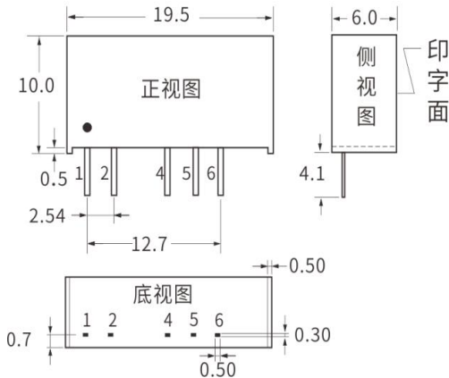
1) 外观尺寸(单位:mm公差:xx ±0.25)
