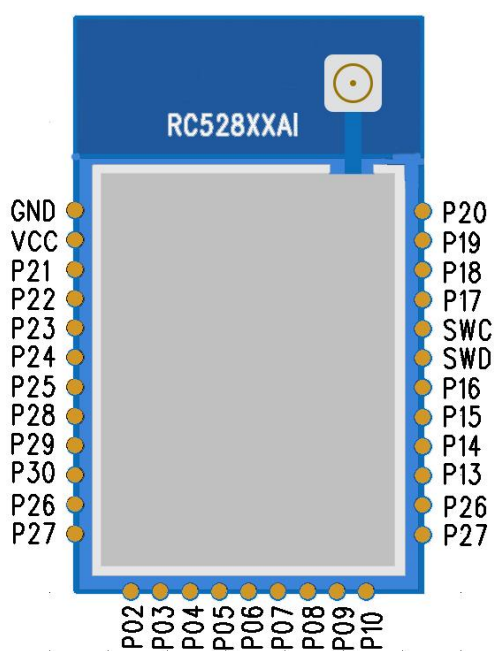
RC52810AI 模块引脚图
