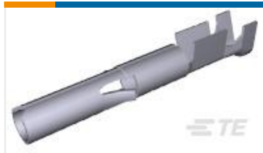
TE Part #350689-7 UMNL SOK 24-18 AU BR L/P
