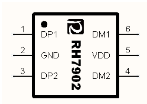
图 1 引脚示意图
