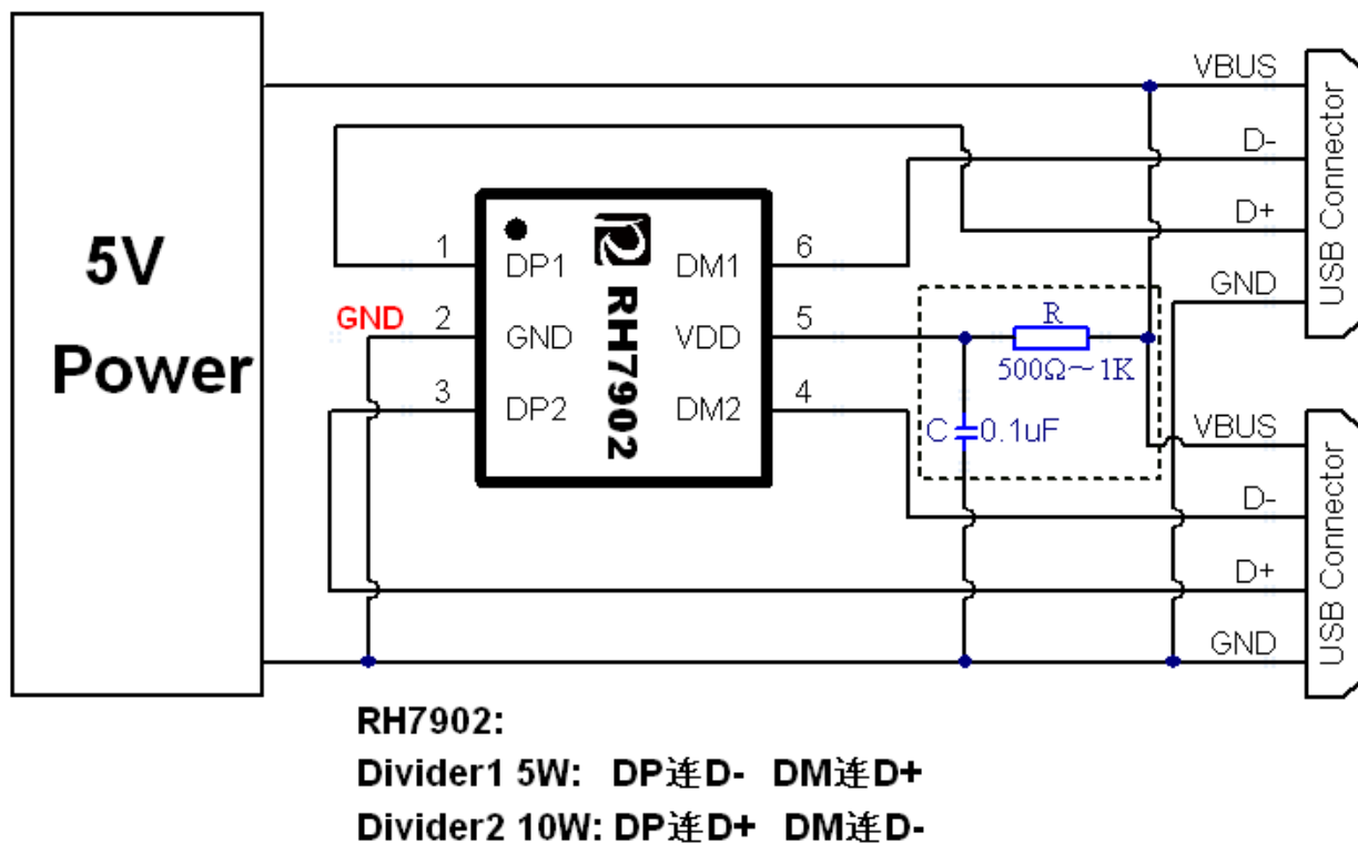
图 3 RH7902电路示意图
