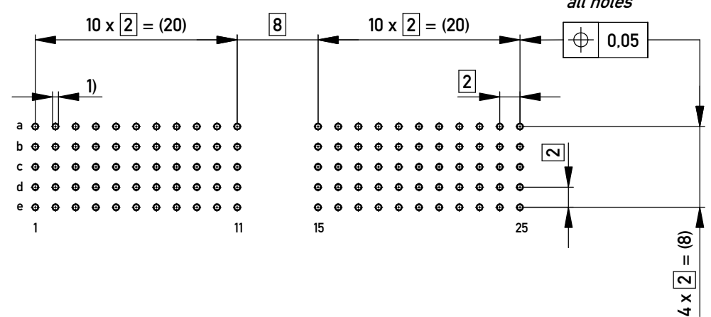
alle Löcher / all holes
