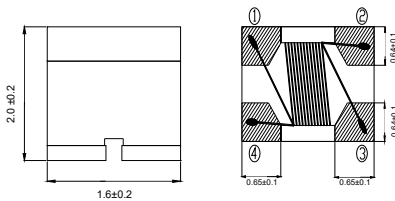
Dimension : mm
