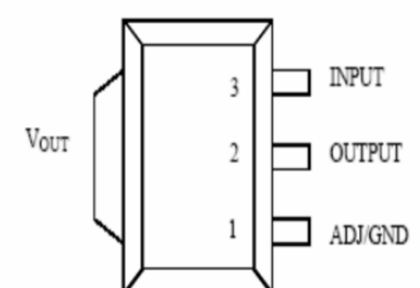
SOT89-3
