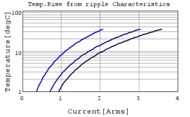
GRM033R61A105ME44 Temp.rise — 100kHz —
