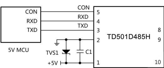
图 3.MCU 5V供电应用电路
