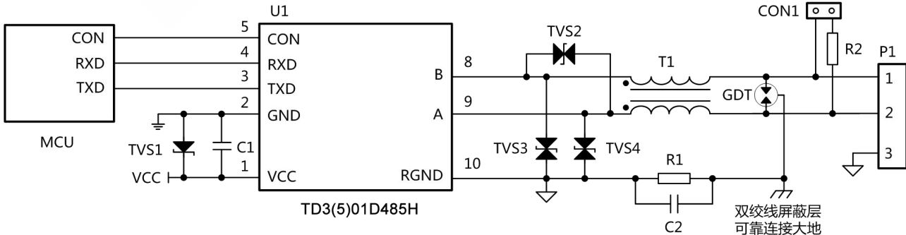
图 5. EMC 推荐电路
