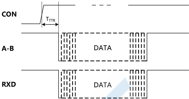
图 2. TD3(5)01D485H模块数据接收时序图
