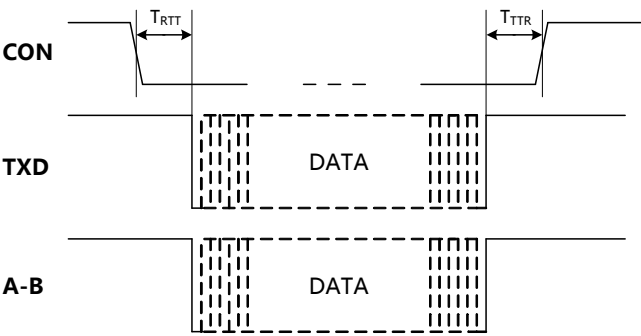
图 1. TD3(5)01D485H模块数据发送时序图
