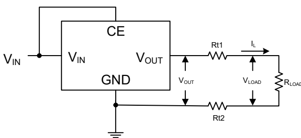
图1. 典型应用电路图
