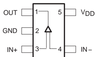
TLV2631 SOT23-5
