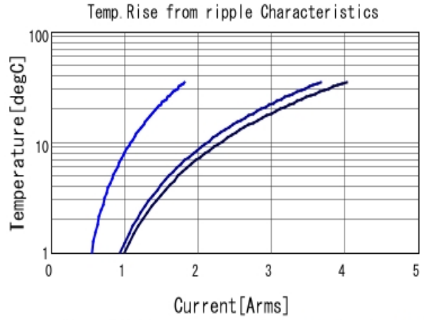
■ GCM21BR71E105KA56 Temp. rise ■ 100kHz ■ 500kHz ■ 1MHz
