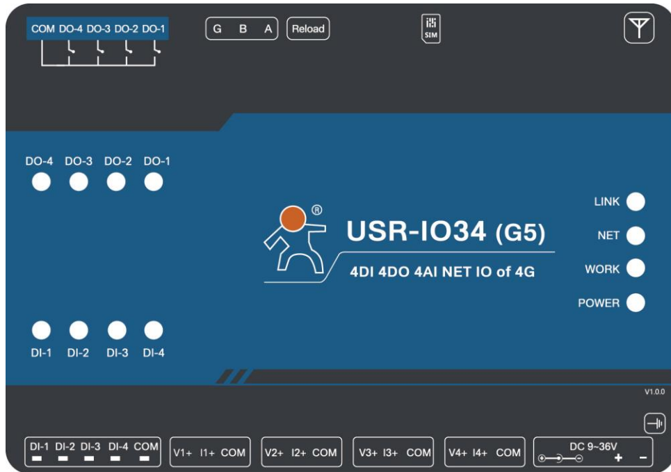
图 13 硬件接口示意图
