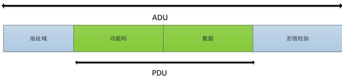
图 32 Modbus RTU 帧
