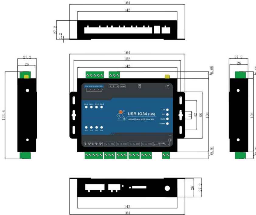
图 14 USR-IO34-G5 尺寸图
