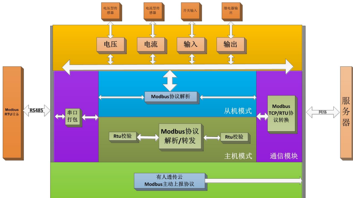
图 15 USR-IO34-G5 功能框图
