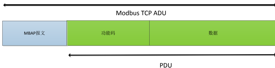
图 33 Modbus TCP 帧
