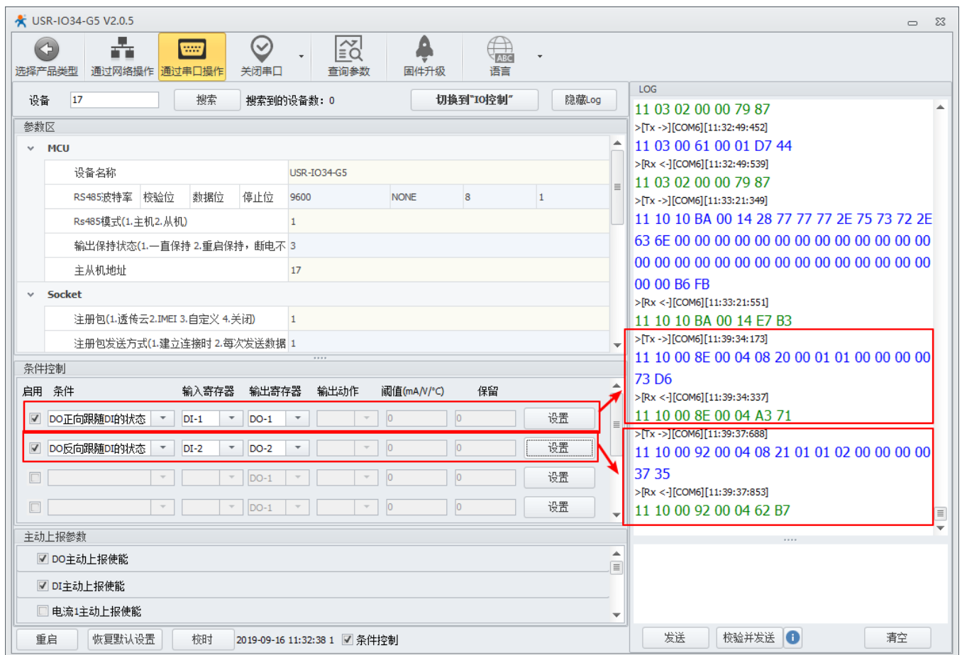
图 20 条件控制操作界面图
