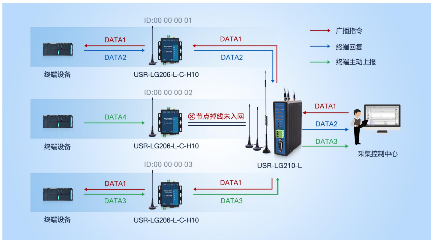
图 2.18 通信过程
