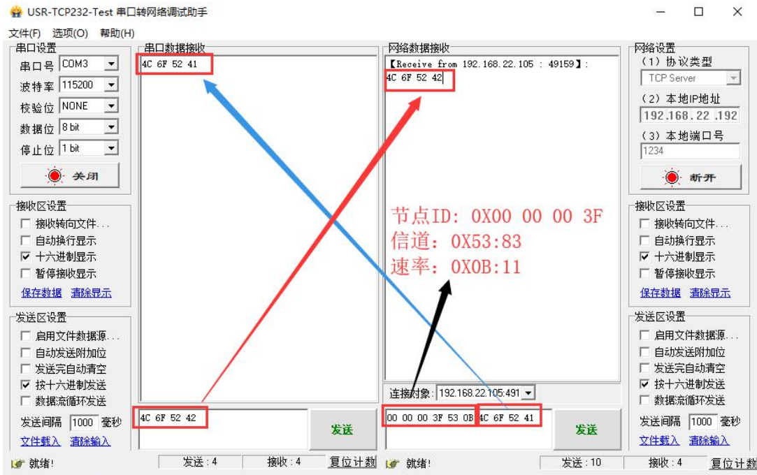
图 2.17 通信过程
