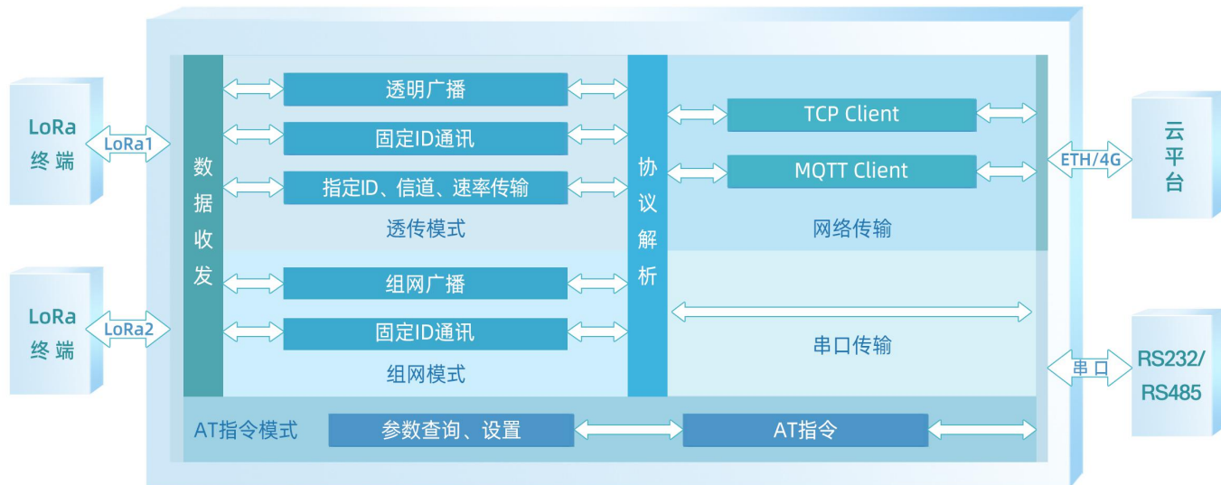
图 2.1 功能框架图
