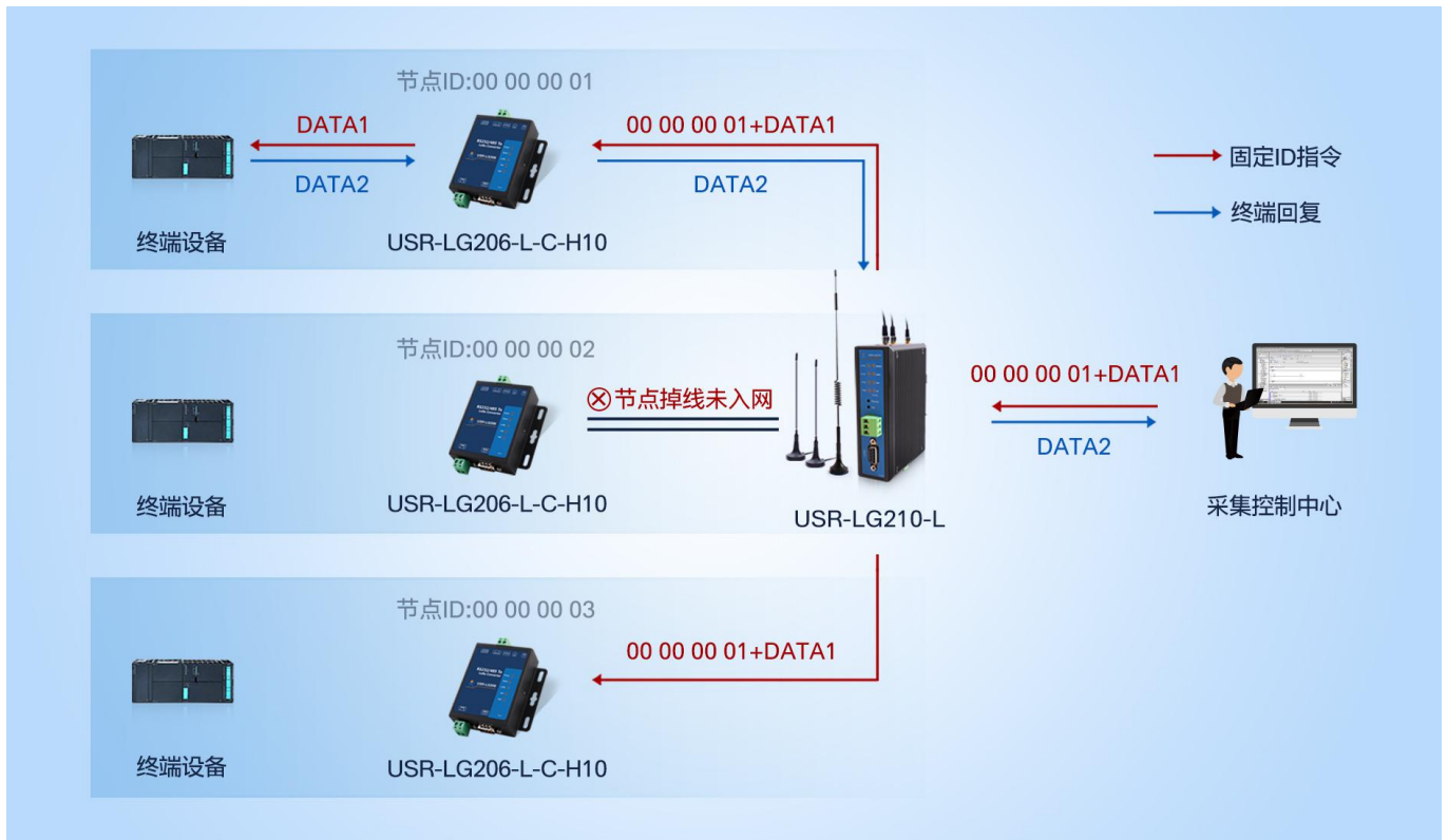
图 2.22 通信过程
