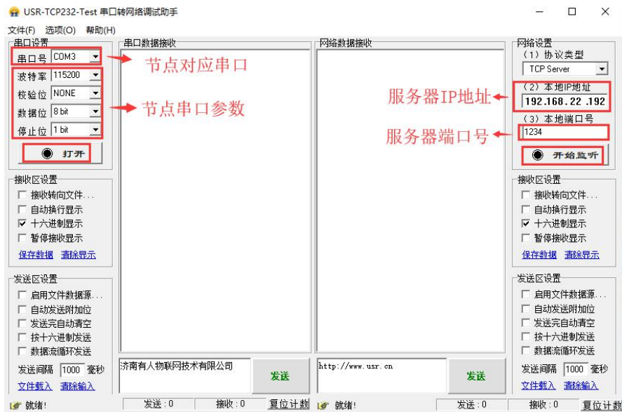
图 2.6 配置示意图
