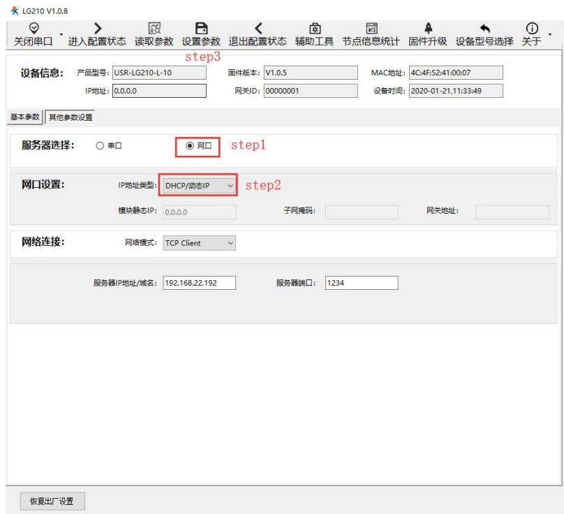
图 3.5 开启 DHCP
