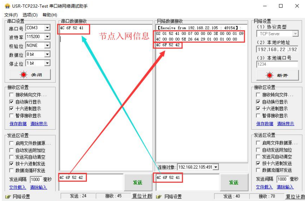
图 2.21 通信过程
