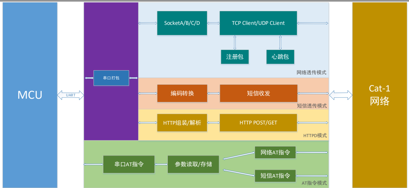
图3. 功能框图
