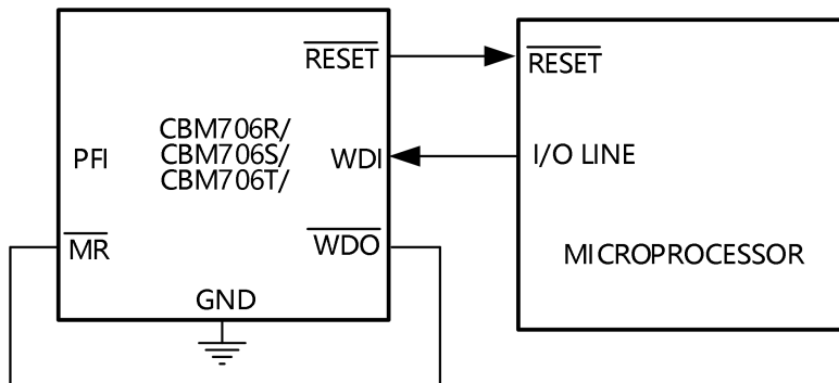
图 21. WDO 的复位
