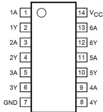
图 3、74HC04引脚排列图
