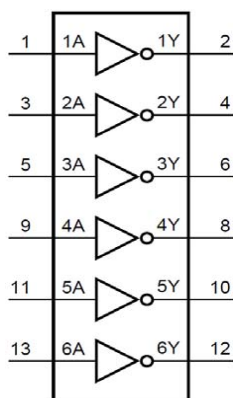
图 1、整体功能框图
