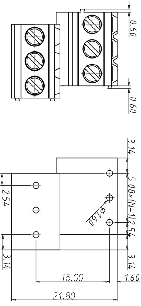
剖面图 A-A
